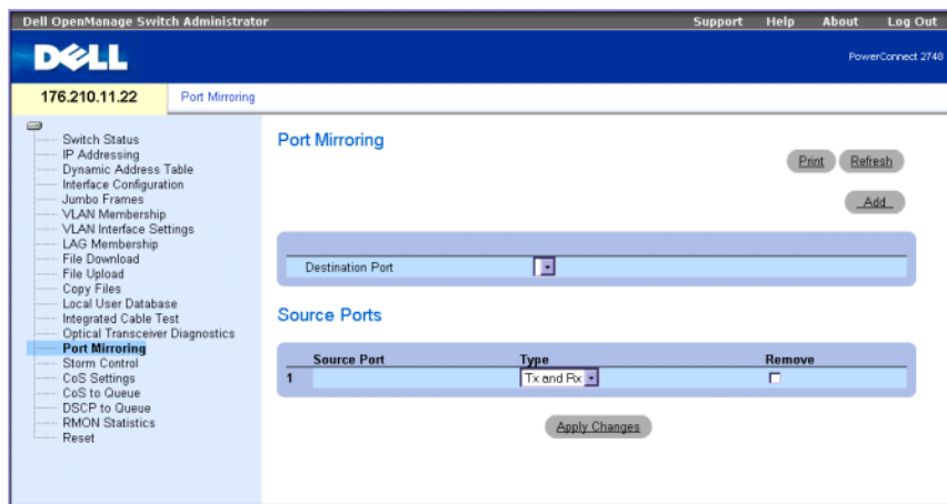
Рисунок 6-15. Зеркалирование портов
