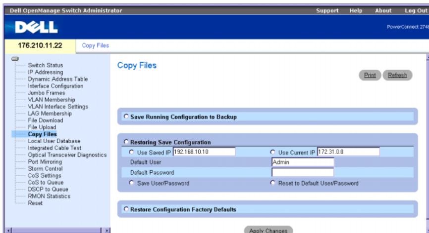
Рисунок 6-11. Копирование файлов
